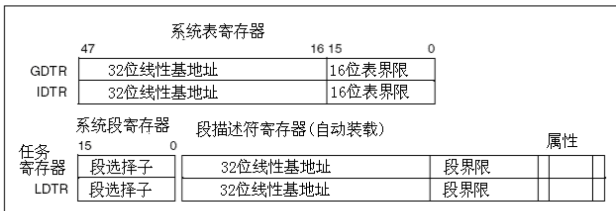
图2-4 内存管理寄存器
